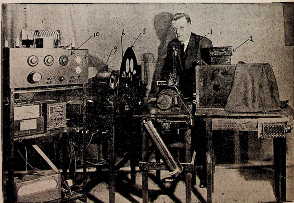
Fig. II. Experimenteele zender met Von Mikaly in het midden.
