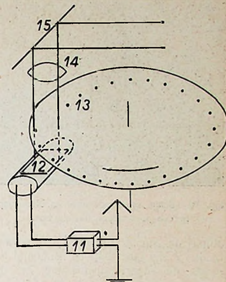
Fig. IV. Schematische voorstelling van den filmtelevisie-ontvanger.
