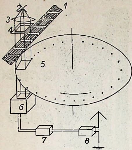
Fig. III. Schematische voorstelling van den filmtelevisie-zender.
