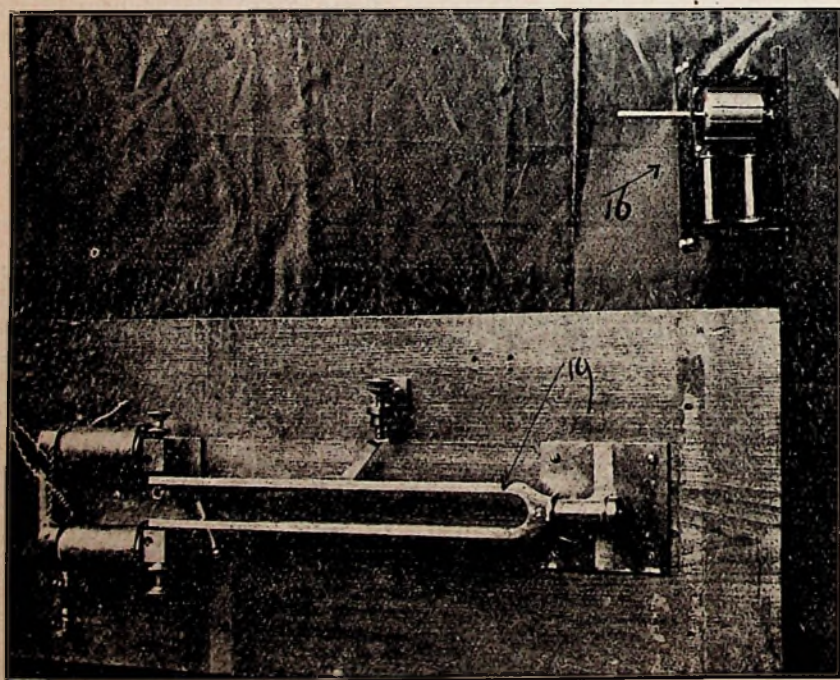
Fig. VII. Synchronomotor (rechts boven) en stemvork als wisselstroomgenerator (onder).
